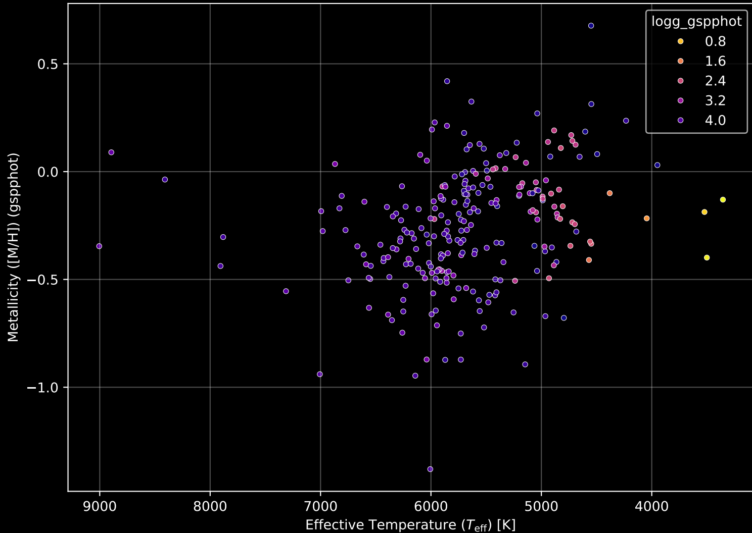
GALAH DR4 Field: [7202] Stellar Population Parameters (n= 247)
