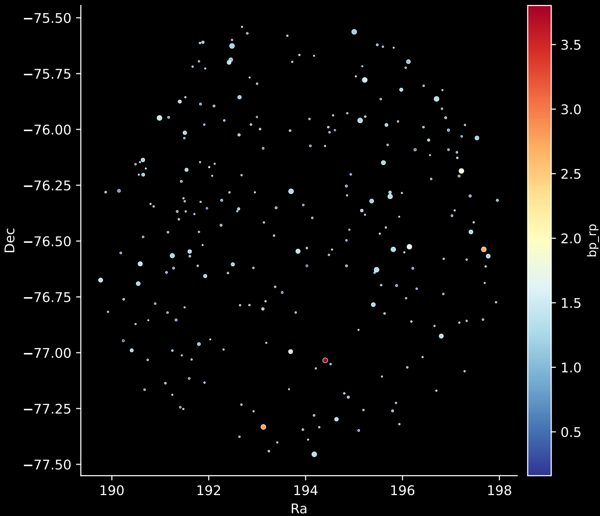
GALAH DR4 Field: [7202] Stars: 247
